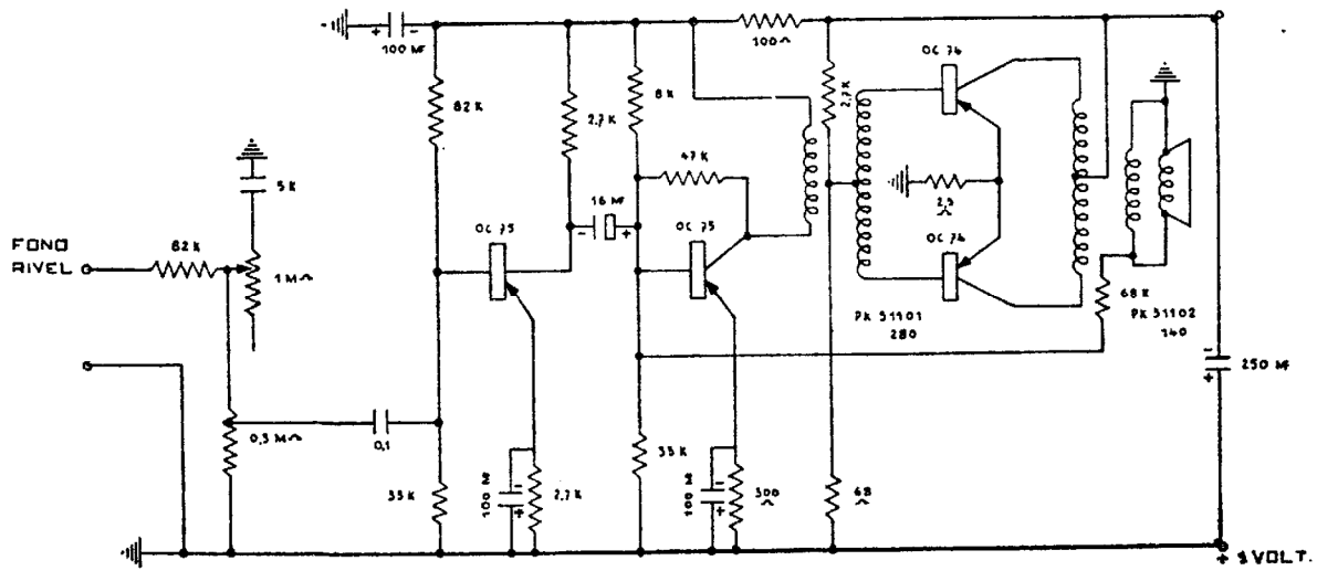
TRANSISTORFONO
